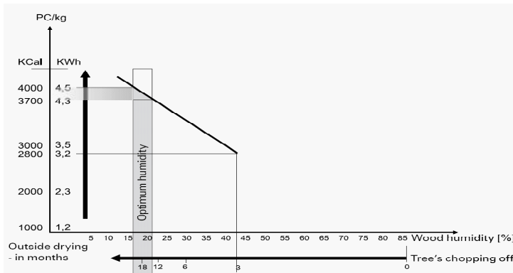
Bild 7. Holzfeuchtigkeit-Diagramm.
